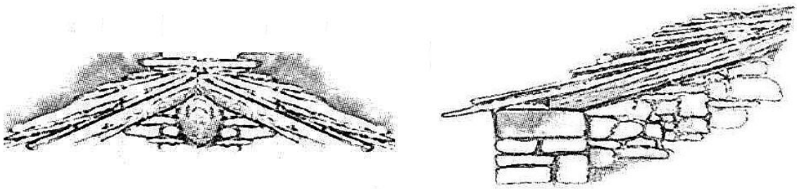
Particolari della copertura da realizzare in scaglie di pietra non segata o 'ciappe'
