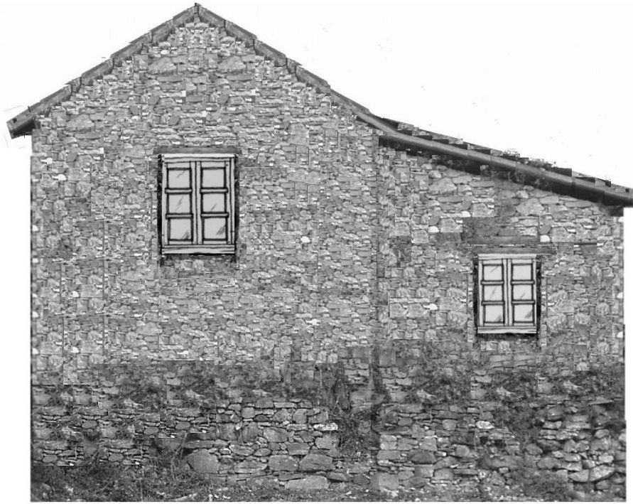
Studio per il restauro della costruzione rurale che ospiterà il museo dell'antica arte olearia - lato ovest
